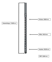
Plastifizier-Schnecke
