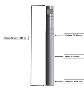
Plastifizier-Zylinder
