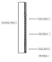
Plastifizier-Schnecke
